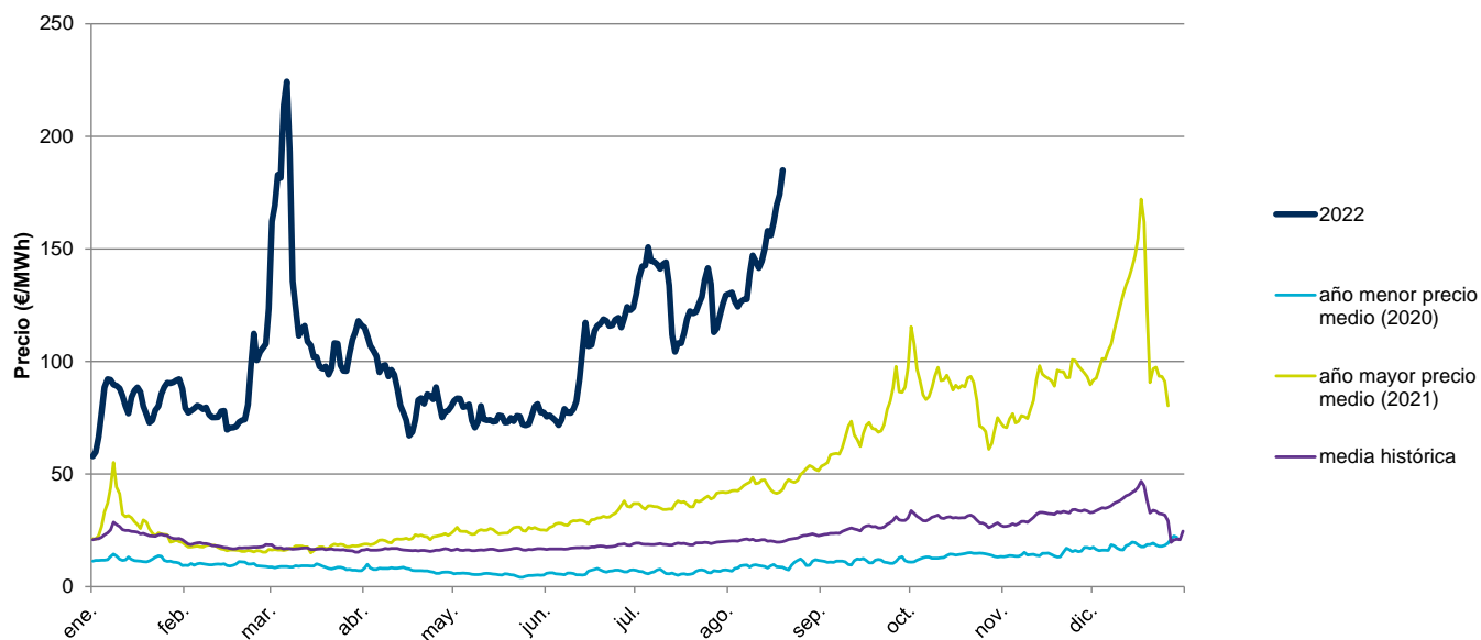
Índice MIBGAS - 2022
